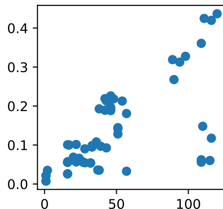
avx
