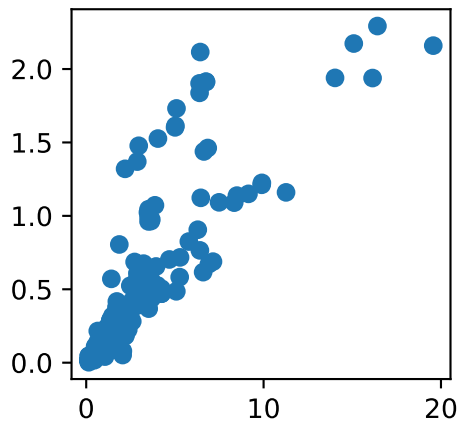
vdt
