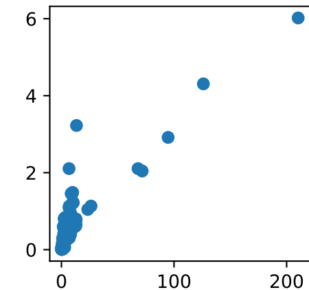
fdlibm
