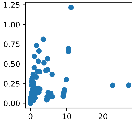
numpy
