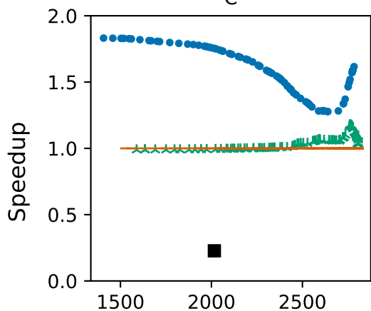
vdt
