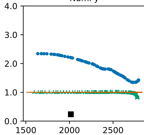
NumPy
