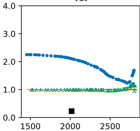
vdt
