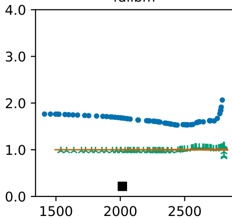
fdlibm
